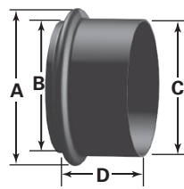
Marmon Flange P235796 P235797
